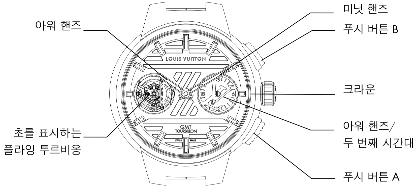
LV 82 칼리버
