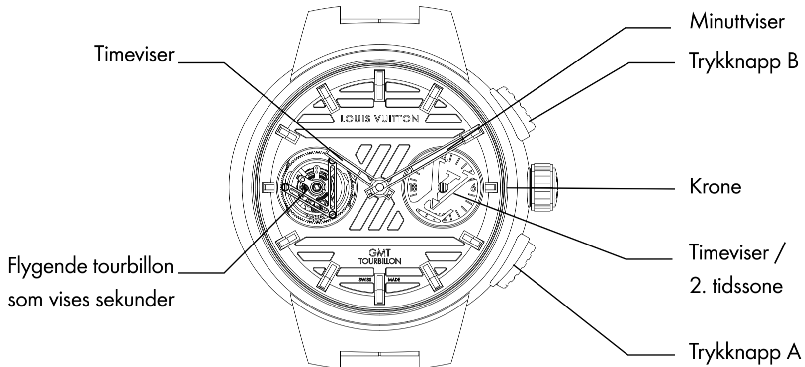
Calibre LV 82
