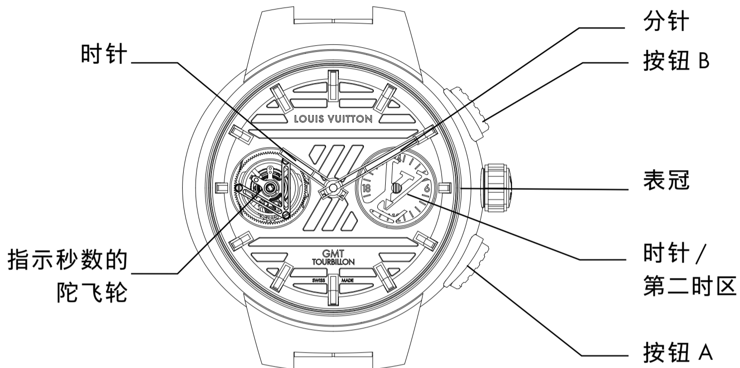
LV 82 机芯
